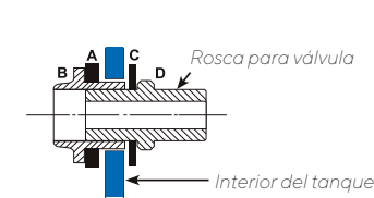
1. Conexión de entrada \varnothing 1/2"
