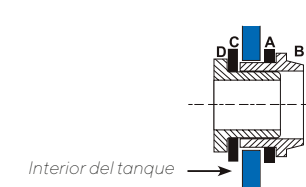
3. Conexión de rebose \varnothing 1"
