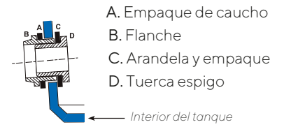
2. Conexión de salida al servicio \varnothing 1"
